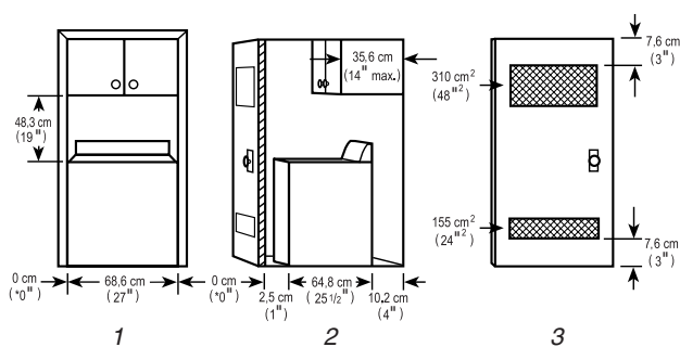
1. Vista frontal 2. Vista lateral 3. Puerta del armario con celosías de ventilación
